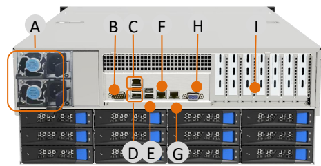
A: 1+1冗余电源×2 B: COM口 C: IPMI端口 D: USB 2.0×2 E: USB 3.0×2 F: LAN1 G: LAN2 H: VGA接口 I: PCI-E扩展插槽
